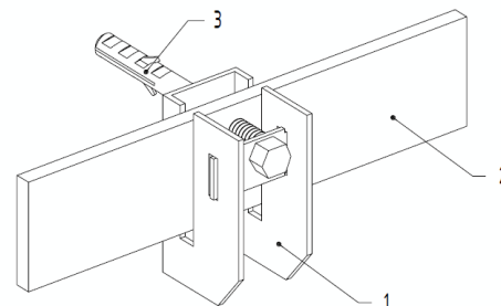
1 - держатель 2 - полоса до 8 мм толщиной 3 - крепление на стену
