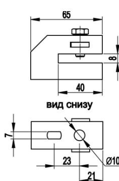
1 - держатель 2 - полоса до 8 мм толщиной 3 - крепление на стену
