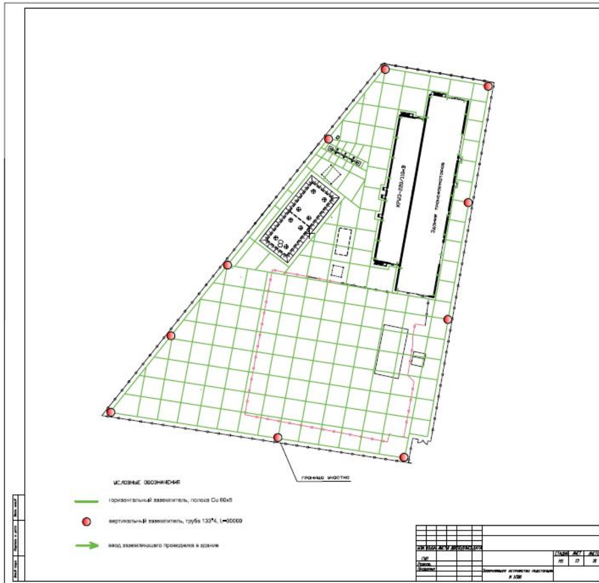
Рис.П.Д.2. Схема наружного заземляющего устройства закрытой ПС с КРУЭ-220 кВ и КРУЭ-110 кВ, переходным пунктом 220 кВ
